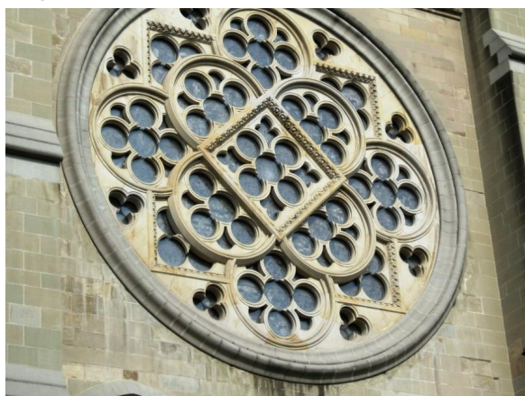
Zone inférieure du cercle de la Rose. Remplacement des Assises jusqu'à la moitié de l'épaisseur des murs en Maçonnerie.
