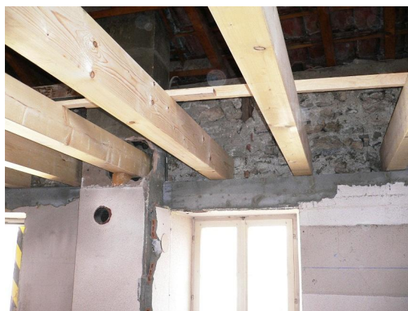
Nouveau plancher bois
