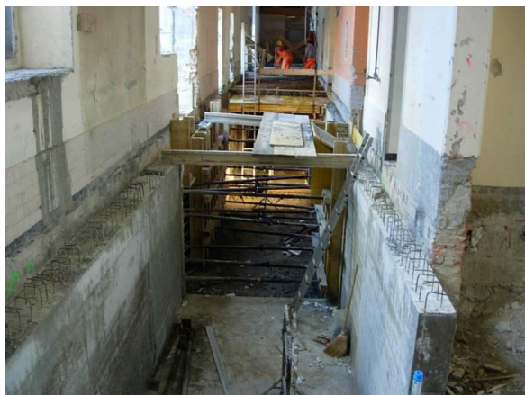
Galerie technique réalisée en sous-œuvre sur toute la Longueur du bâtiment
