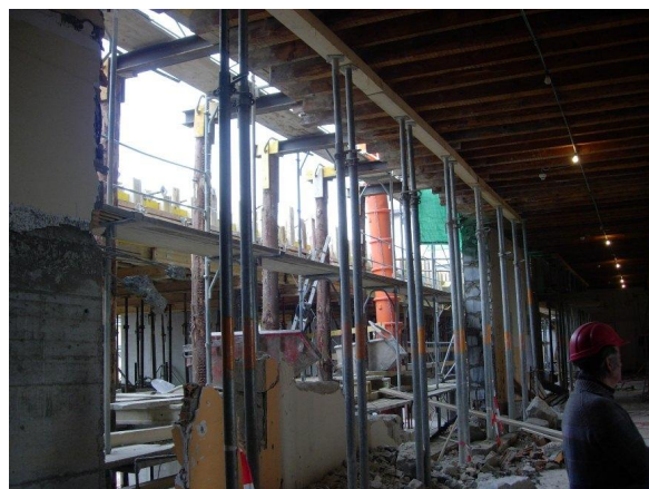
Création d'ouverture dans la façade existante
