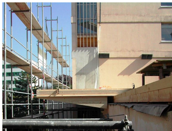
Plancher avec console pour porte-à-faux
