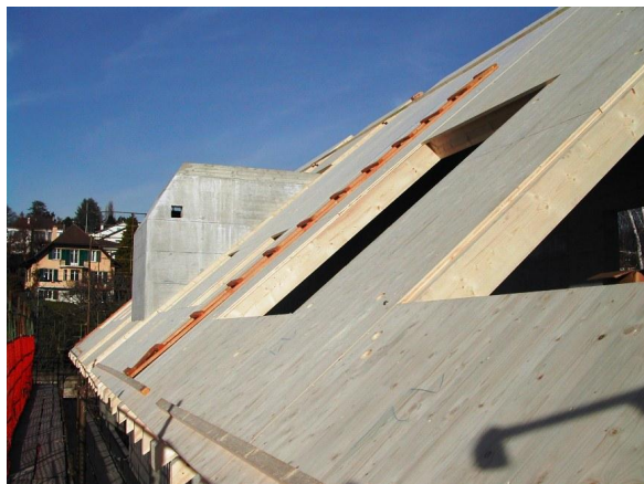
Toiture bois préfabriquée
